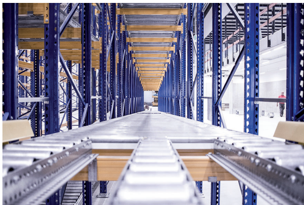
Durchlaufregal im neuen Lagergebäude in Neuenburg.
